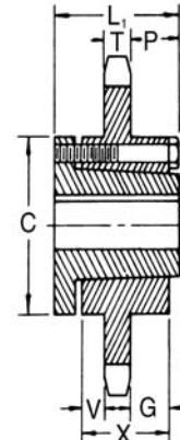
PD — TIPO C 1
