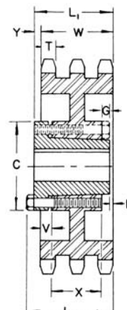
QD — TIPO B1
