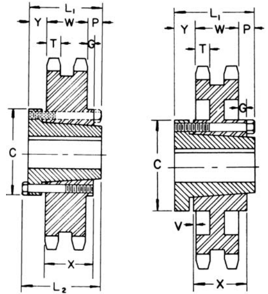
QD — TIPO C 2
