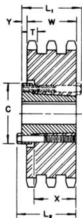
QD — TIPO B
