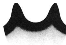
Parte Endurecida del Diente
