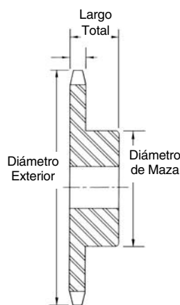
Sencillo Maza Tipo B
