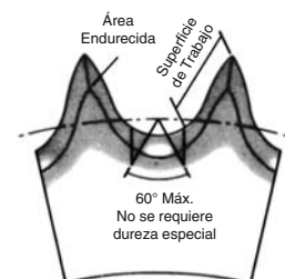
Profundidad de la Dureza Requerida
